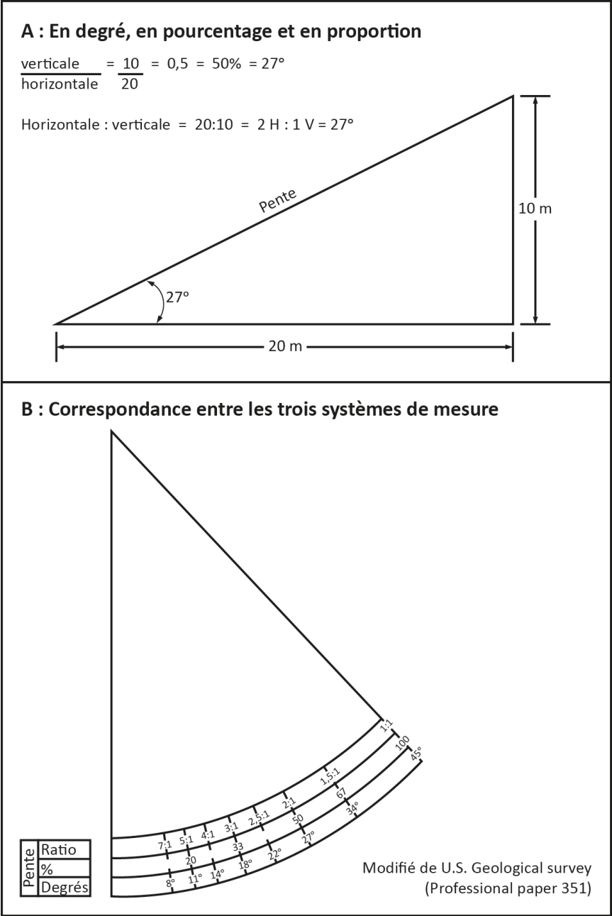
Figure 29. Illustrations des diverses façons d'exprimer une inclinaison
