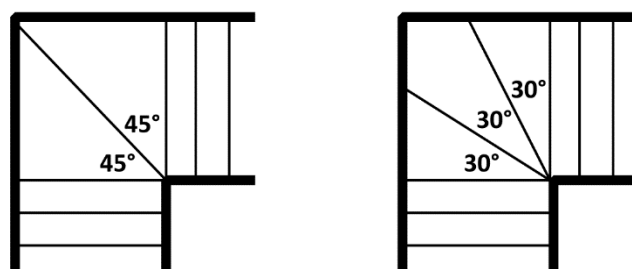
Figure 28 : Marches rayonnantes
